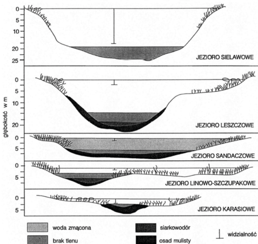
Rys. 3. Schemat rybnych typów jezior
